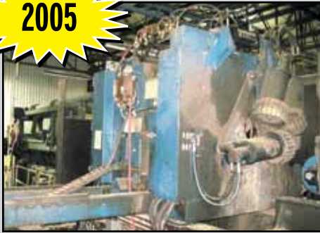
FORANO CAMBIO MT-451-94-A9 18" RING DEBARKER
