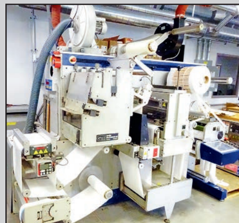
GRAFISK MASKINFABRIK DC330-MINI E LABEL FINISHING MACHINE
